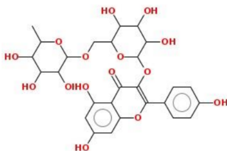
Gambar 1. Struktur kimia senyawa kampferenol
