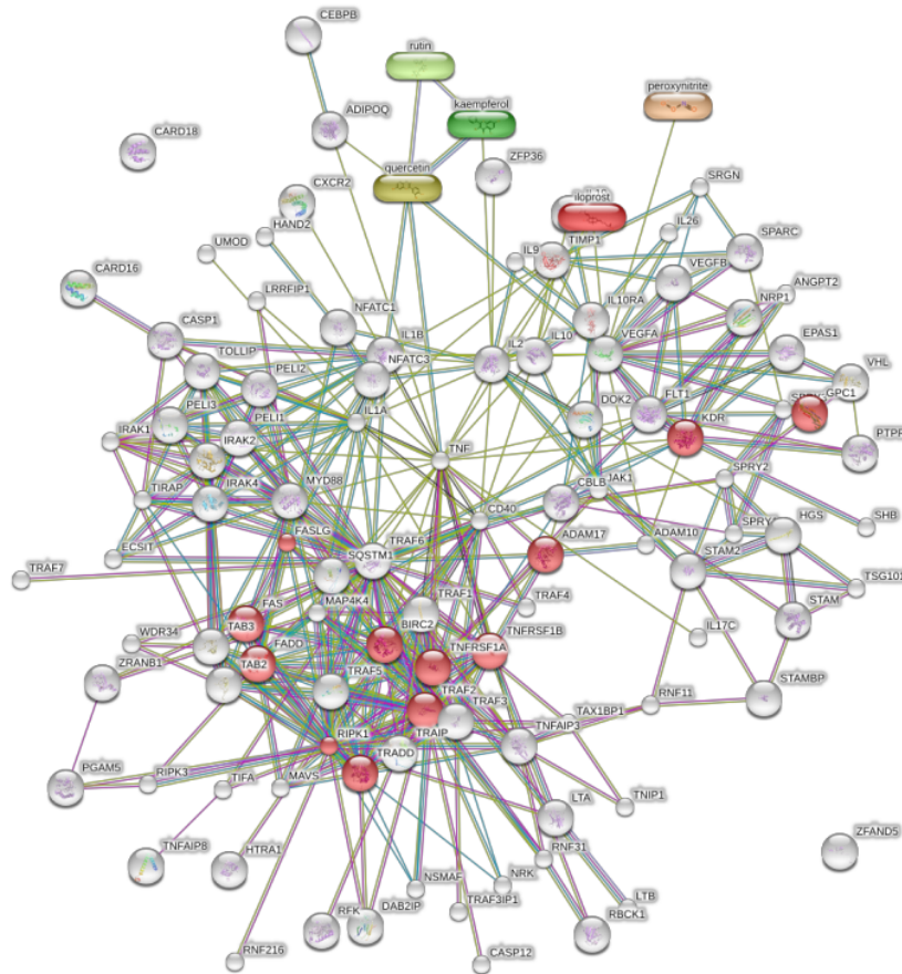
Gambar 4. Mekanisme regulasi senyawa pada kandungan carica pubescens terhadap peningkatan proliferasi, diferensiasi dan immunorespon
