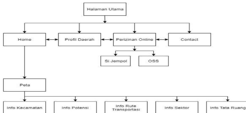
Gambar-3 Struktur Navigasi Web SIG
