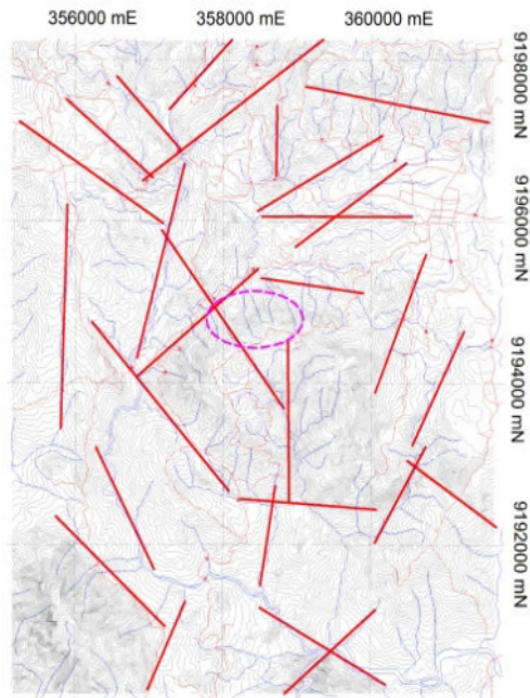
Gambar 5. Kelurusan struktur geologi pada peta topografi daerah penelitian dan sekitarnya.
