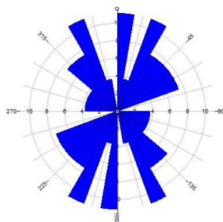
Gambar 6. Diagram bunga Kelurusan struktur geologi daerah penelitian
