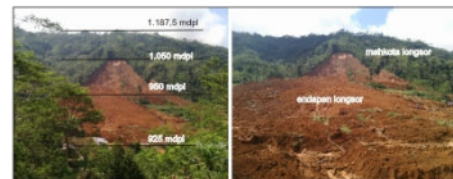
Gambar 3. Morfologi lereng longsor di daerah penelitian
