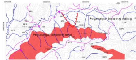
Gambar 2. Peta Geomorfologi daerah penelitian
