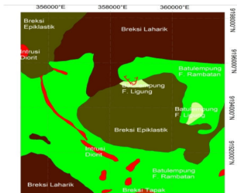
Gambar 1. Peta Geologi Regional daerah penelitian (Condon, dkk., 1996).
