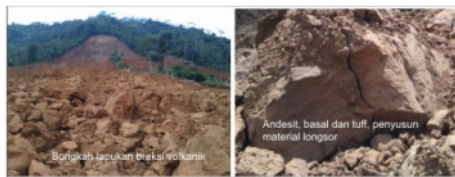
Gambar 4. Bongkah lapukan batuan dan fragmen batuan yang masih segar di daerah penelitian
