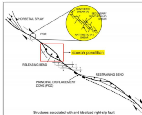
Gambar 8. Model konseptual sesar di daerah penelitian [15].
