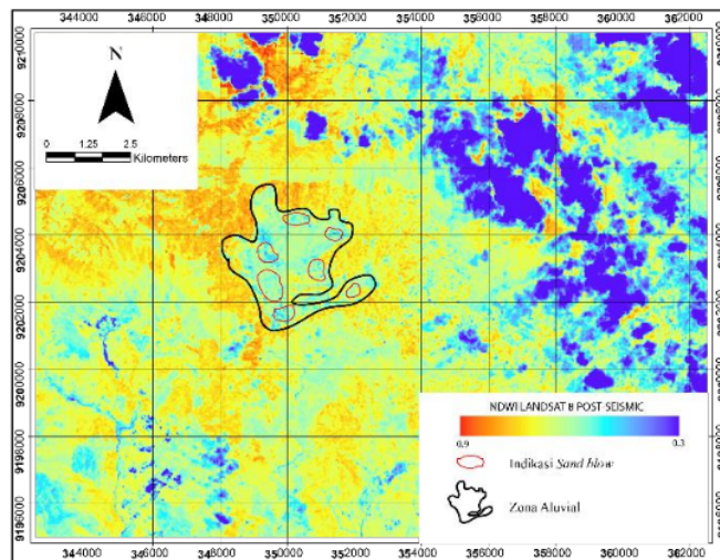
Gambar 10. Peta NDWI Kalibening sesudah terjadi gempa.
