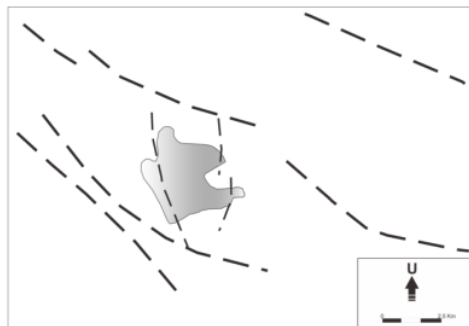
Gambar 7. Hasil interpretasi pola struktur geologi daerah penelitian.
