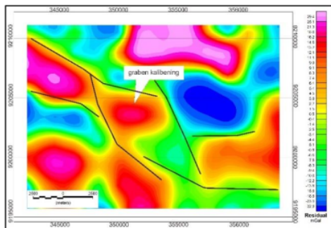
Gambar 6. Peta anomali gaya berat.
