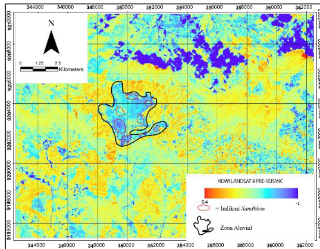
Gambar 9. Peta NDWI Kalibening sebelum terjadi gempa.
