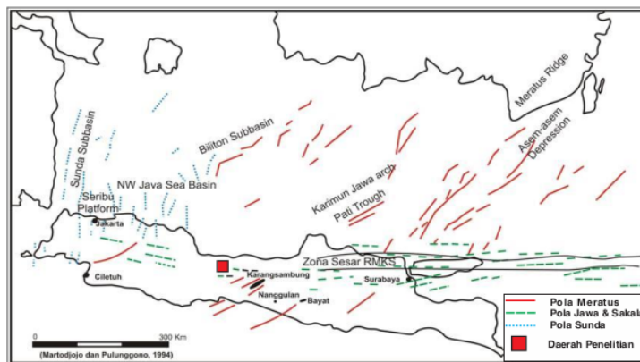
Gambar 3. Pola struktur Pulau Jawa [12].
