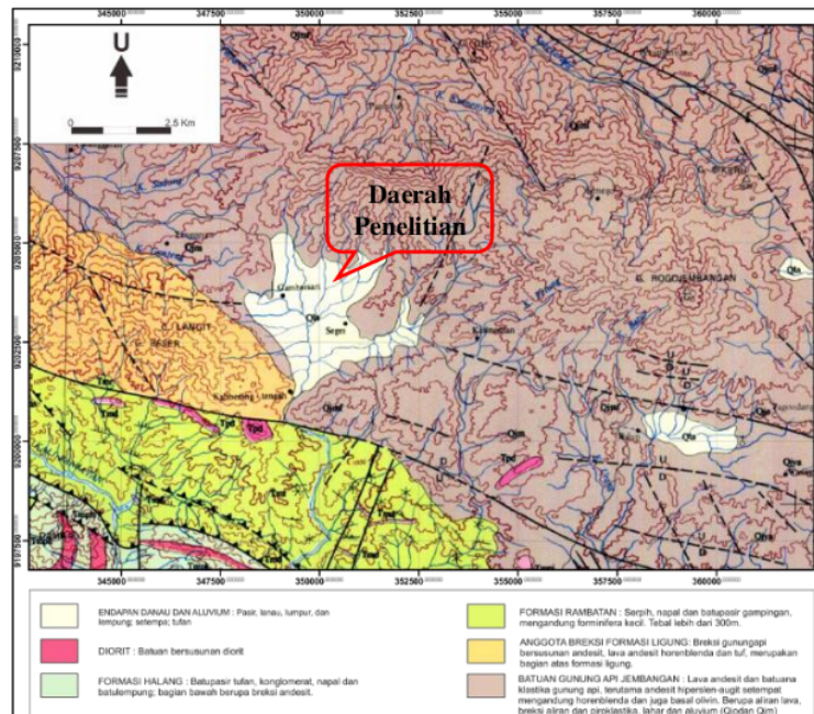
Gambar 1. Modifikasi peta geologi regional Banjarnegara-Pekalongan [9].
