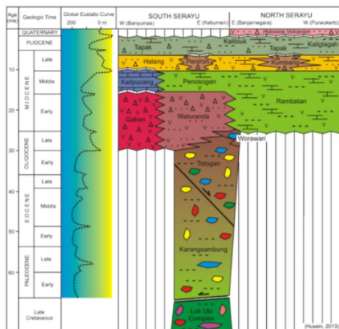
Gambar 2. Kolom stratigrafi regional daerah penelitian [10], [11].
