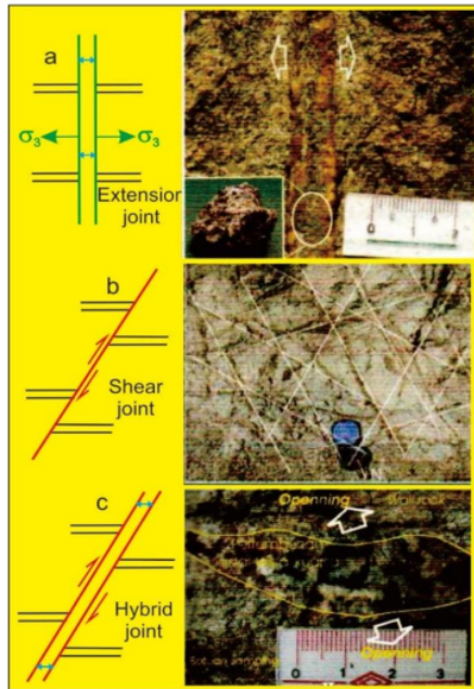
Gambar 9. Jenis-jenis kekar (Mc Clay, 2007) dan contoh di daerah penelitian
