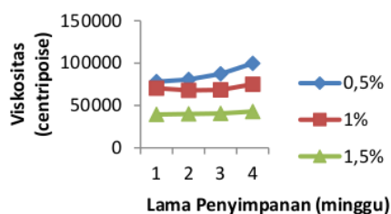
Gambar 1 Hubungan antara lama penyimpanan dengan viskositas
