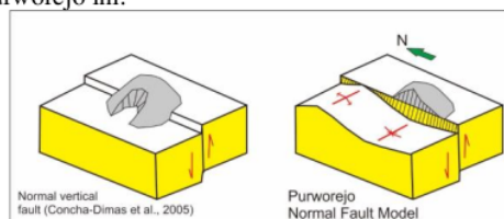
Gambar 8. Diagram pengaruh sesar normal terhadap bentuk gunung api [15] serta kondisi di jalur sesar Purworejo
