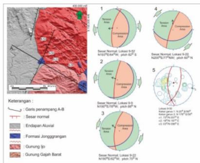
Gambar 4. Analisis data gores-garis dan kekar pada jalur sesar ekstensional Purworejo.
