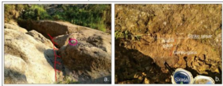
Gambar 3. Kenampakan lapangan sesar normal Purworejo di Desa Plipir Kecamatan Purworejo.
