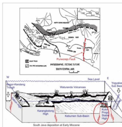
Gambar 7. Sesar Normal Purworejo menurut [2].
