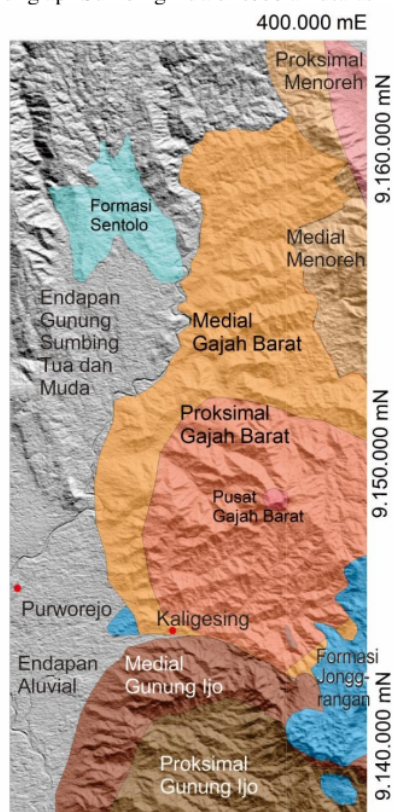
Gambar 6. Fasies medial Gunung Gajah Barat melampar luas ke arah utara namun terpotong dan hanya sempit di arah barat
