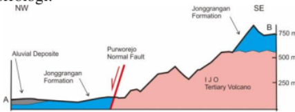
Gambar 5. Penampang geologi dari garis penampang A-B pada Gambar 4.
