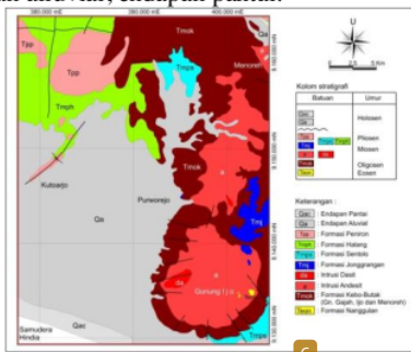
Gambar 2. Tatanan stratigrafi regional daerah penelitian menurut peta geologi regional lembar Yogyakarta [9] dan peta geologi lembar Kebumen [4]
