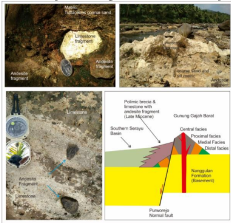
Gambar 9. Breksi polimik di Purworejo-barat Pegunungan Kulon Progo yang tidak dijumpai di Pegunungan Kulon Progo. Semua batuan tersebut menumpang diatas Formasi nanggulan sebagai batuan dasar daerah penelitian
