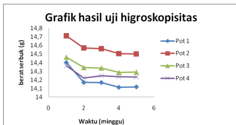
Gambar 4. Grafik hasil uji higroskopisitas.
