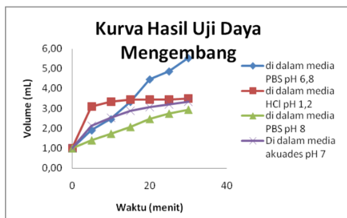
Gambar 6. Kurva hasil uji daya mengembang tepung agar.
