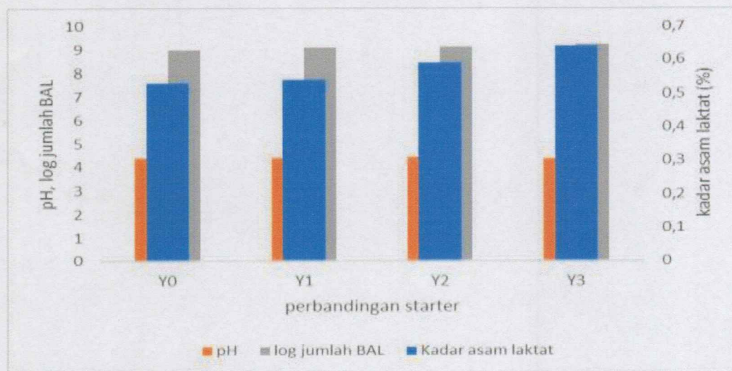
Gambar 1. Histogram rata-rata kadar asam laktat, pH, dan log jumlah Bakteri Asam Laktat pada yoghurt hasil fermentasi L. bulgaricus dan S. thermophilus dengan penambahan Bifidobacterium Bb2E (Y0 2:2:0, Y1 2:2:1, Y2 2:2:2, Y3 2:2:3)
