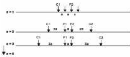
Gambar 2. Pergerakan elektroda arus dan potensial pada saat akuisisi data tahanan jenis dengan konfigurasi Schlumberger.
