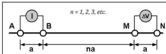
Gambar 3. Susunan dan jarak antar elektroda pada akuisisi data resistivitas menggunakan konfigurasi dipole-dipole.
