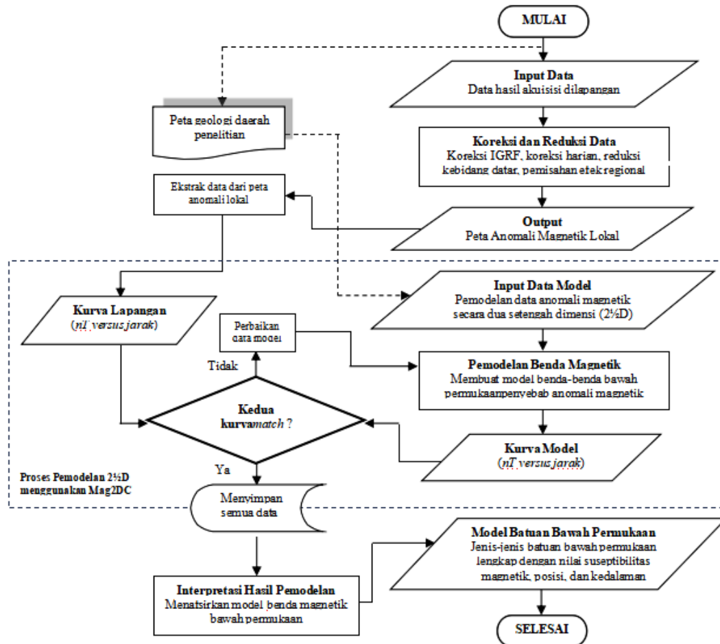
Gambar 4: Diagram alir sistematika pengolahan data anomali magnetik; pengolahan, pemodelan, dan interpretasi data anomali magnetik.
