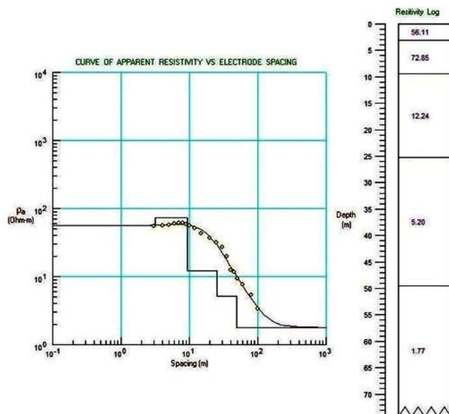
Gambar 8: Hasil pemodelan resistivitas batuan bawah permukaan di titik Sch-03.
