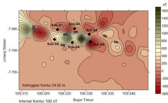
Gambar 5: Plotting titik-titik sounding di atas peta kontur anomali magnetik lokal dalam survey geolistrik resistivitas.
