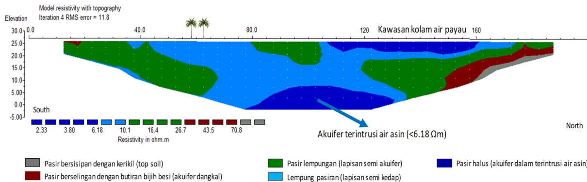
Gambar 12 Profil litologi batuan bawah permukaan 2D pada lintasan NWT-04 yang menunjukkan bagian akuifer yang terintrusi air asin (saltwater)
