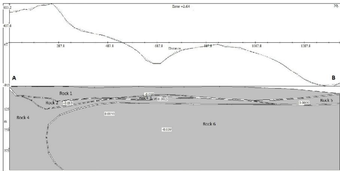
Gambar 6. (color online) Hasil pemodelan menggunakan software Mag2DC for Window terhadap data-data pada lintasan AB (panjang lintasan adalah AB 1433,62 meter)
