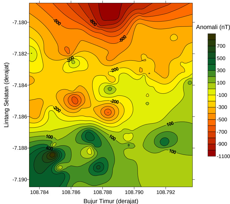
Gambar 2. (color online) Peta kontur anomali medan magnetik total daerah penelitian (interval kontur 100nT).
