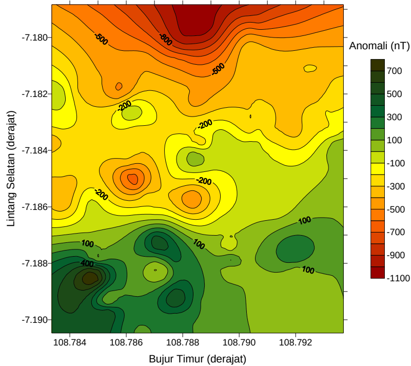
Gambar 3. (color online) Peta kontur anomali magnetik total yang telah direduksi ke bidang datar (interval kontur 100nT).
