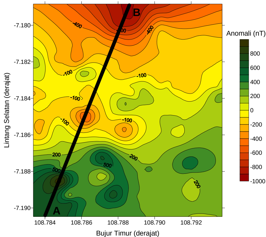
Gambar 5. (color online) Peta kontur anomali medan magnetik lokal daerah penelitian dan lintasan pemodelan AB (interval kontur 100nT)
