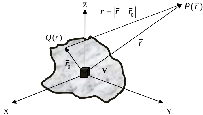
Gambar 1. (color online) Potensial magnetik pada titik P di permukaan bumi akibat distribusi massa termagnetisasi yang kontinu di bawah permukaan
