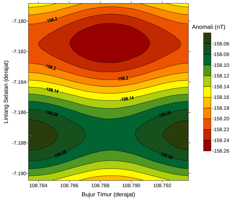
Gambar 4. (color online) Peta kontur anomali magnetik regional daerah penelitian
