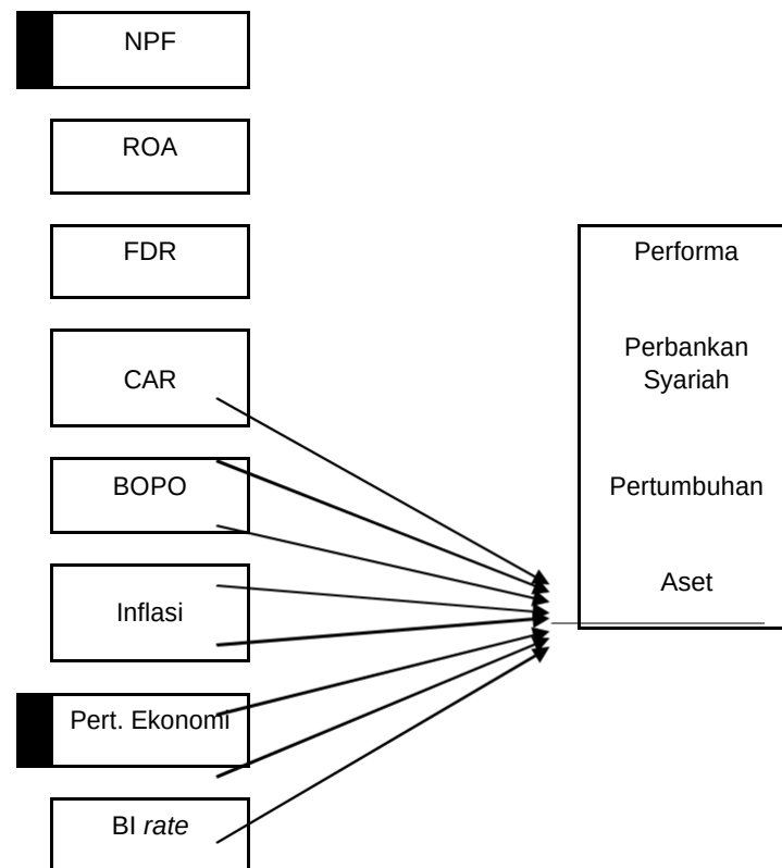
Gambar 2. Kerangka Pemikiran
