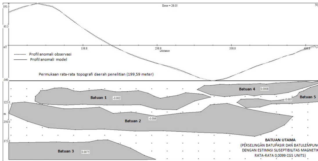
Gambar 6. Hasil pemodelan anomali magnetik menggunakan perangkat lunak Mag2DC for Window pada sayatan CD.
