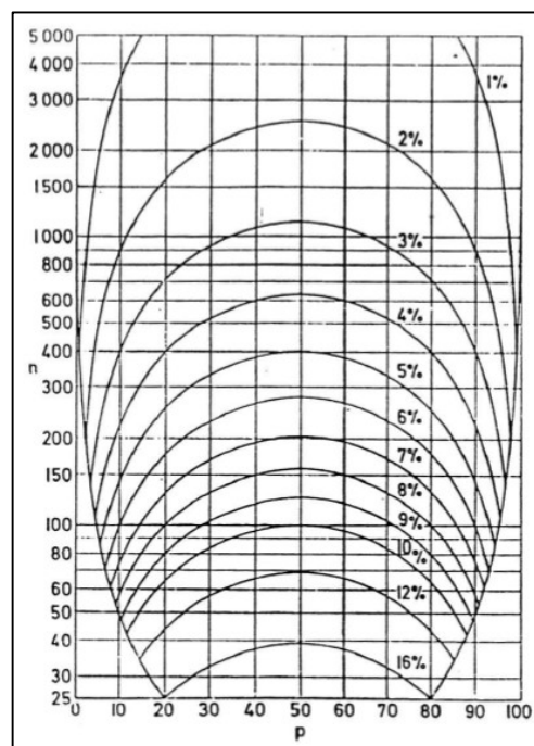
Gambar 2. Diagram Van der Plas yang digunakan untuk mencari nilai simpangan baku mineral berat. Simbol n = jumlah total mineral yang dihitung, p = persentase setiap mineral. Misalnya: n = 300 , p = 25\% , maka simpangan bakunya adalah 5%. Sehingga persentase mineral yang dihitung antara 20%-30%. Dalam hal ini nilai p + simpangan baku yang diambil, sehingga p terkoreksi 30% (Rohendi dan Aryanto, 2016; Setyanto dan Surachman, 2017)
