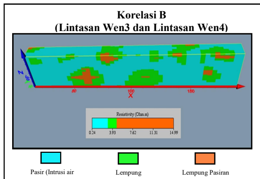
Gambar 16. Korelasi Lintasan Wen3 dan Lintasan Wen4 dalam bentuk penampang resistivitas 3D
