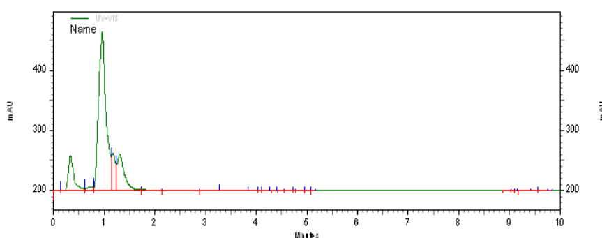
Gambar 4. Kromatogram dari senyawa triadimefon dalam sampel air sungai
