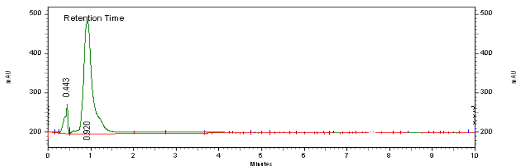
Gambar 3. Kromatogram dari standar triadimefon 50 ppm
