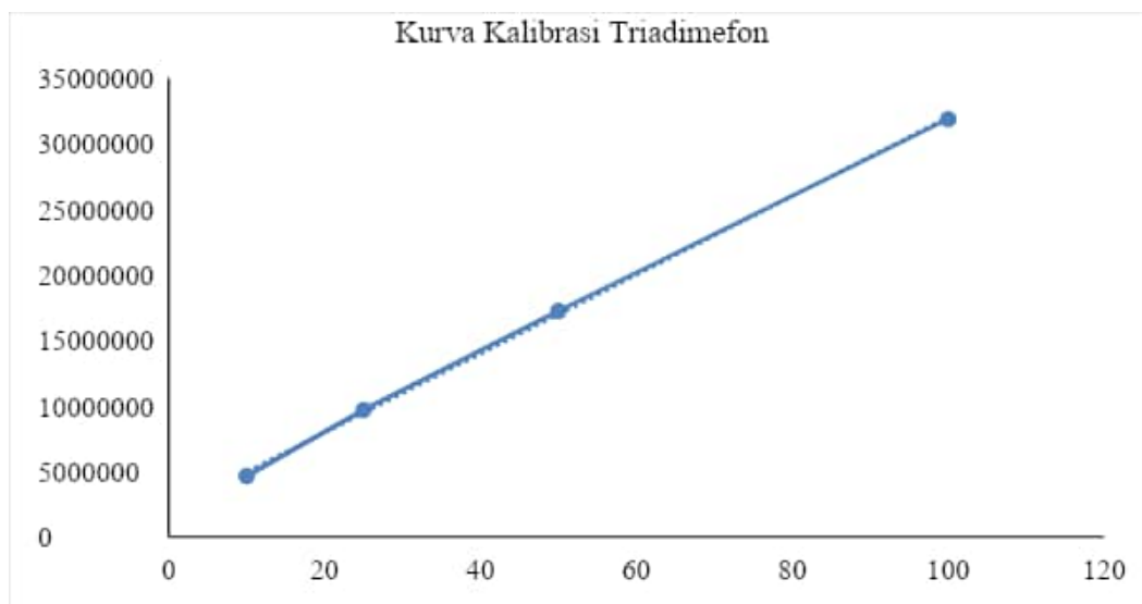
Gambar 2. Grafik hubungan antara konsentrasi standar triadimefon dengan luas area
