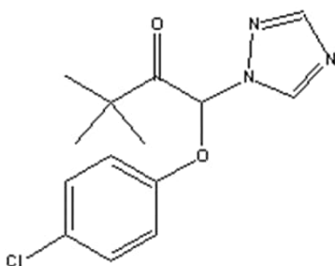
Gambar 1. Struktur kimia dari triadimefon
