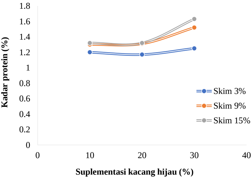
Gambar 7 Kadar protein sari jagung manis yang dipengaruhi suplementasi kacang hijau dan susu skim Sumber: [52]
