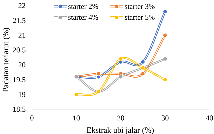
Gambar 16 Total padatan terlarut sari jagung probiotik pada variasi konsentrasi starter dan suplementasi ekstrak ubi jalar Sumber [24]
