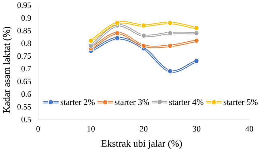
Gambar 14 Kadar asam laktat sari jagung probiotik yang dipengaruhi konsentrasi starter dan suplementasi ekstrak ubi jalar Sumber : [24]
