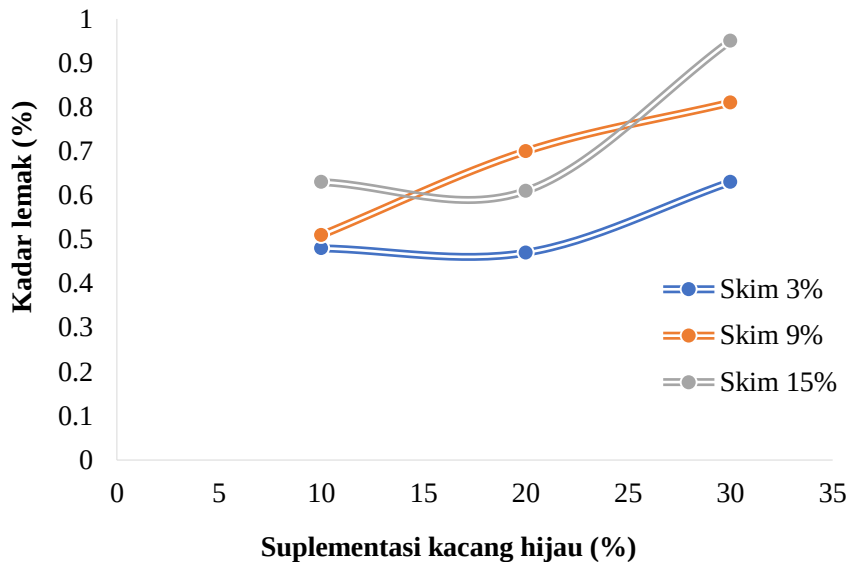
Gambar 6 Kadar lemak sari jagung manis yang dipengaruhi suplementasi kacang hijau dan susu skim Sumber : [55]
