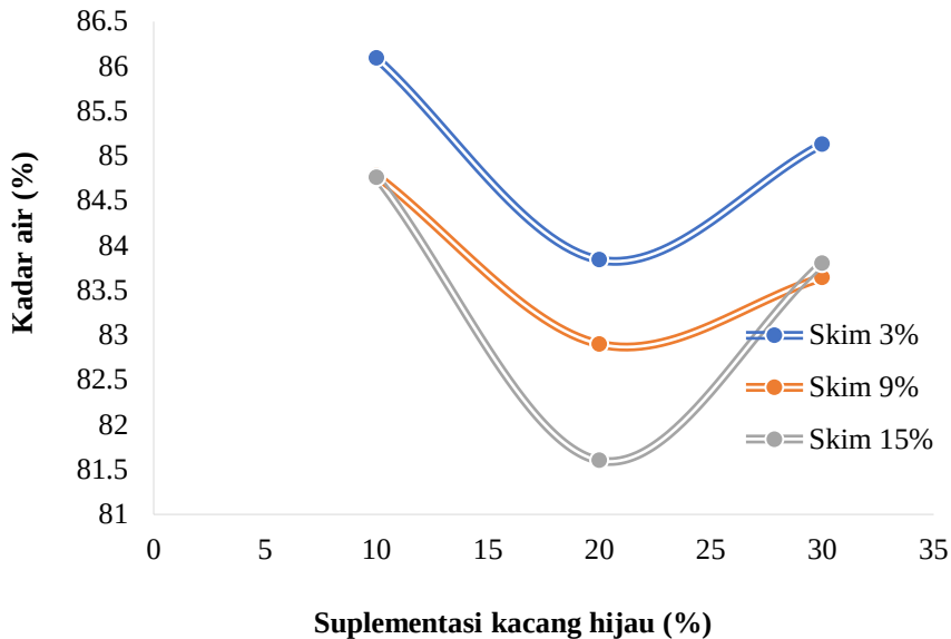
Gambar 5 Kadar air sari jagung manis yang dipengaruhi suplementasi kacang hijau dan susu skim Sumber [52]
