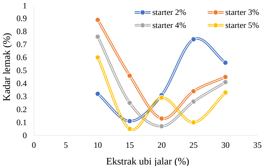
Gambar 11 Kadar lemak sari jagung probiotik yang dipengaruhi konsentrasi starter dan suplementasi ekstrak ubi jalar (Sumber : [24])
