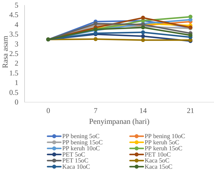
Gambar 26 Rasa asam sari jagung probiotik yang dikemas kaca, polipropilene (PP) dan polietilen terphthalate (PET) selama penyimpanan (Sumber [53],[54])
