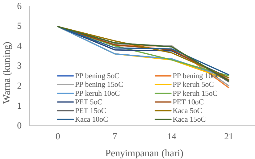
Gambar 24 Warna sari jagung probiotik yang dikemas kaca, polipropilene (PP) dan polietilen terphthalate selama penyimpanan Sumber [53],[54]
