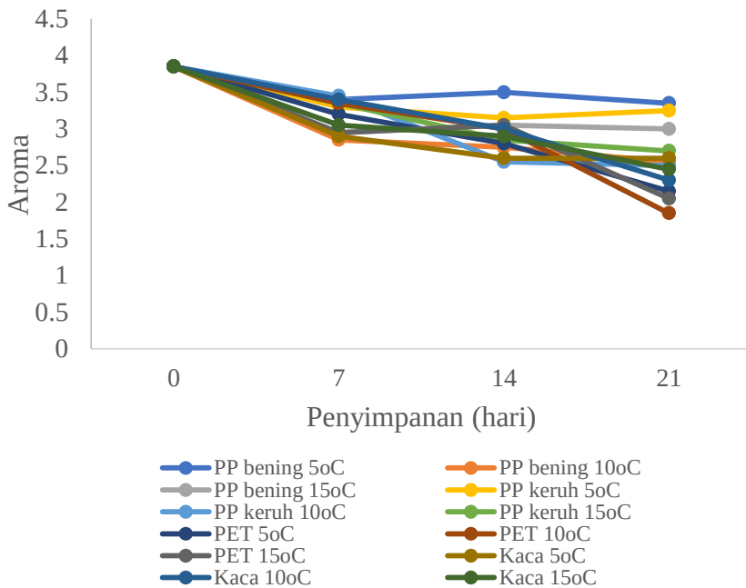
Gambar 25 Aroma sari jagung probiotik yang dikemas kaca, polipropilene (PP) dan polietilen terephthalate (PET) selama penyimpanan (Sumber [53],[54])
