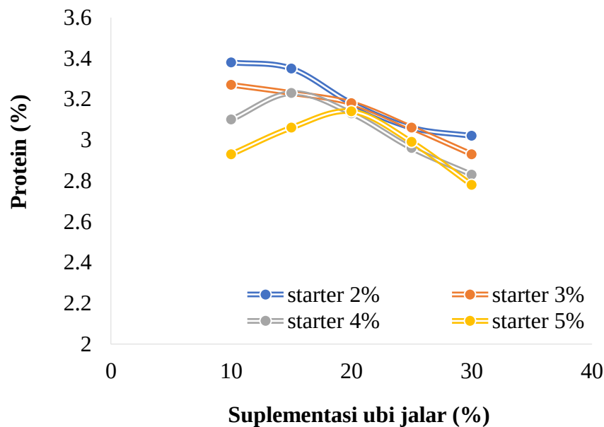
Gambar 12 Kadar protein sari jagung probiotik yang dipengaruhi konsentrasi starter dan suplementasi ekstrak ubi jalar (Sumber : [24])
