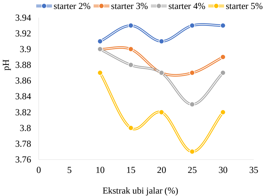
Gambar 15 pH sari jagung probiotik pada variasi konsentrasi starter dan ekstrak ubi jalar Sumber [24]
