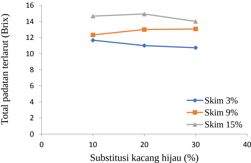
Gambar 3 Total padatan terlarut sari jagung manis dengan variasi substitusi kacang hijau dan penambahan susu skim Sumber [52]
