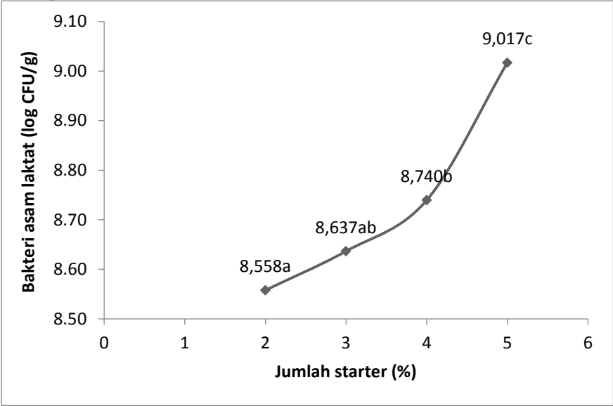
Gambar 10 Jumlah bakteri asam laktat pada sari jagung probiotik Sumber: [24]
