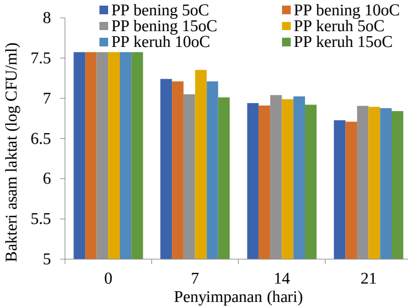
Gambar 18 Jumlah bakteri asam laktat pada sari jagung probiotik yang dikemas botol polipropilene (PP) Sumber [53]
