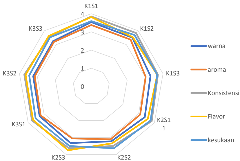
Gambar 8 Sifat sensoris sari jagung yang dipengaruhi konsentrasi kacang hijau dan susu skim Sumber: [57]
