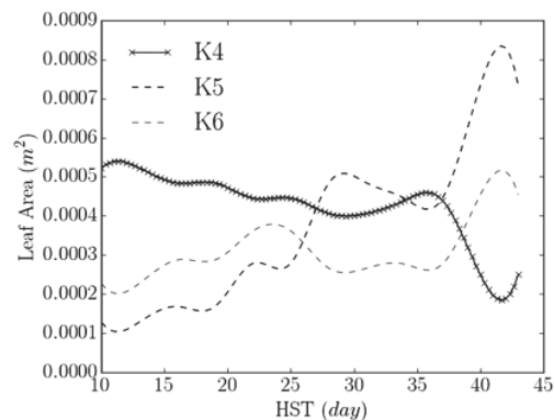
Gambar 4. Pertumbuhan Luas Daun pada Kotak 4, 5, dan 6.
