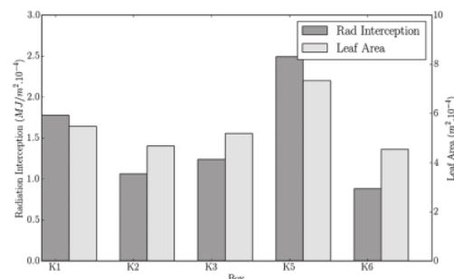
Gambar 5. Luas Daun dan Radiasi Terintersepsi
