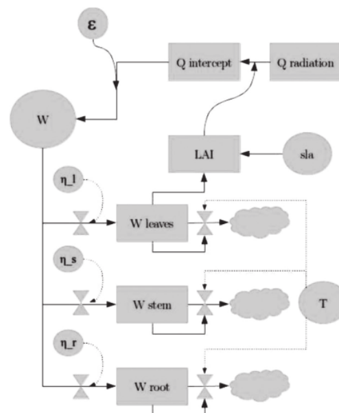
Gambar 2. Bagan Konsep Pertumbuhan dan Perkembangan Biomassa.
