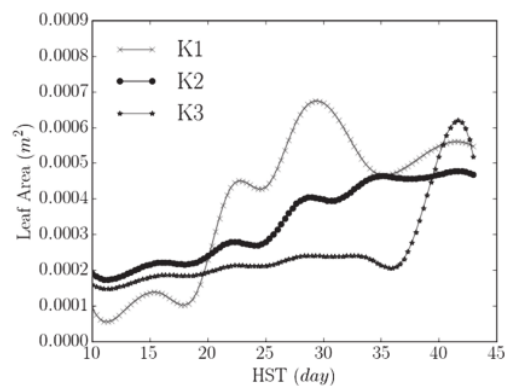
Gambar 3. Pertumbuhan Luas Daun pada Kotak 1, 2, dan 3.
