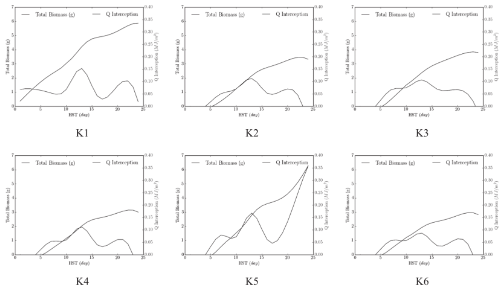
Gambar 6. Simulasi Perkembangan Biomassa dan Radiasi Terintersepsi
