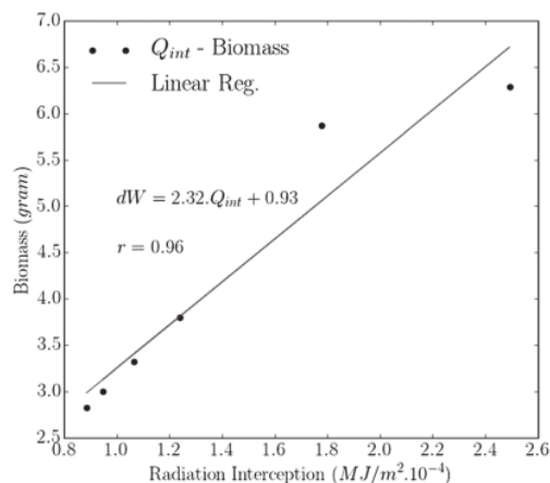
Gambar 7. Simulasi Radiasi Terintersepsi dan Biomassa
