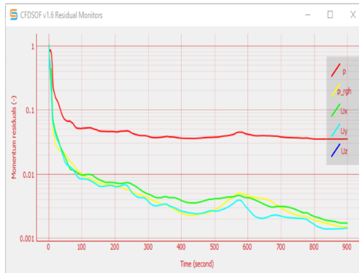
Gambar 8. Proses perhitungan pada CFDSOF.
