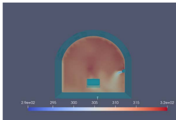
Gambar 11. Kontur temperatur.
