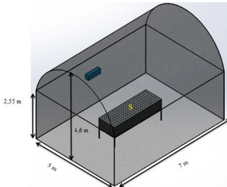
Gambar 3. Greenhouse yang digunakan untuk penelitian
