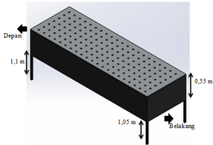
Gambar 1. Layout box aeroponik.
