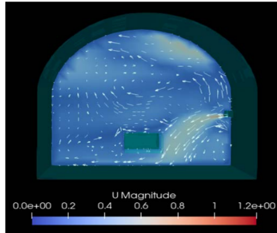
Gambar 12. Vektor Aliran Udara
