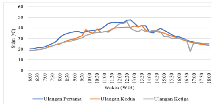
Gambar 4. Distribusi suhu di dalam greenhouse tanpa aplikasi fogging system
