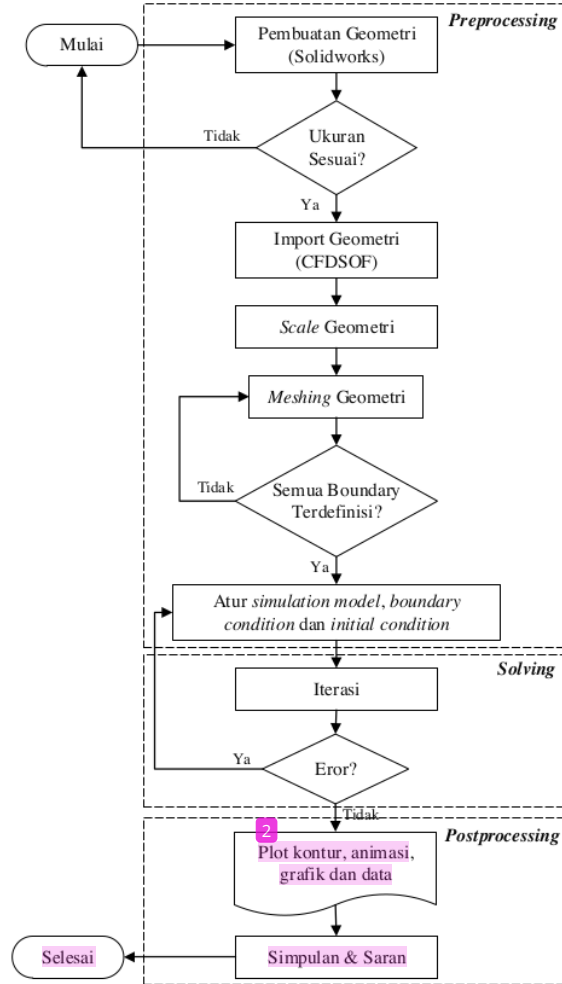
Gambar 2. Diagram alir simulasi CFDSOF.
