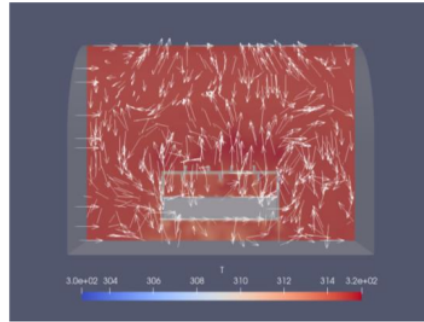
Gambar 8. Hasil vektor suhu udara (tampak sisi).
