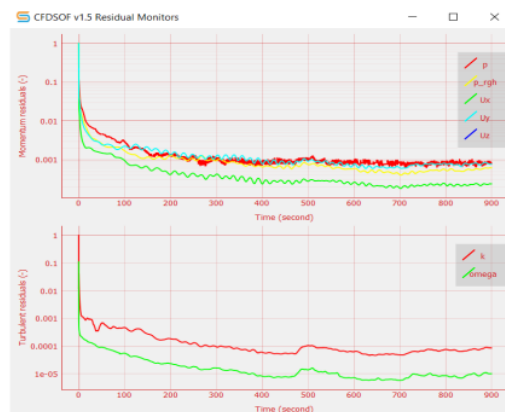
Gambar 7. Proses perhitungan pada CFDSOF.
