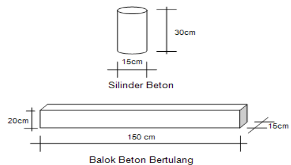
Gambar 1 Benda uji.
