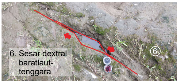
6. Sesar dextral baratlaut-tenggara
