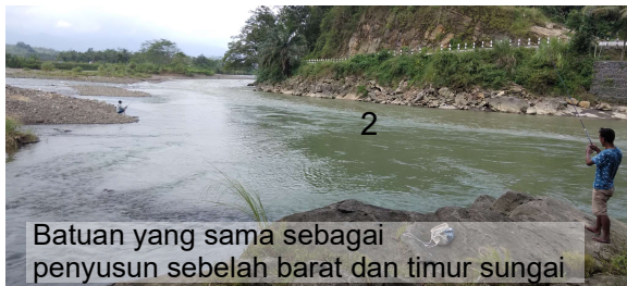
Celah morfologi yang terentuk oleh Sungai Gintung
