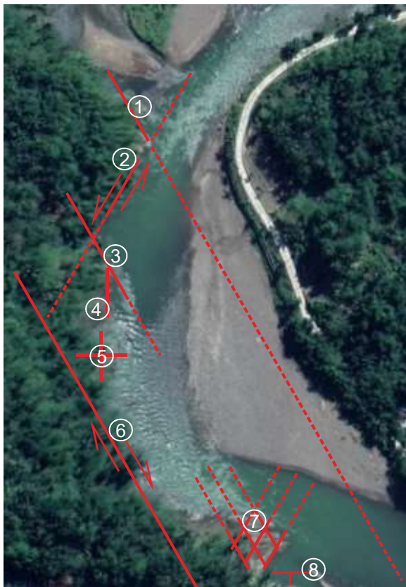
4. Sand dyke berarah utara-selatan
